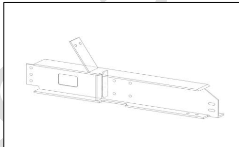
FIGURE 1. SAMPLE PROJECT DRAWING FOR METAL FABRICATOR (FITTER) COMPETITION 2018/EXEMPLE PROJET DESSIN POUR MONTEUR/SOUDEUR CONCURRENCE 2018
